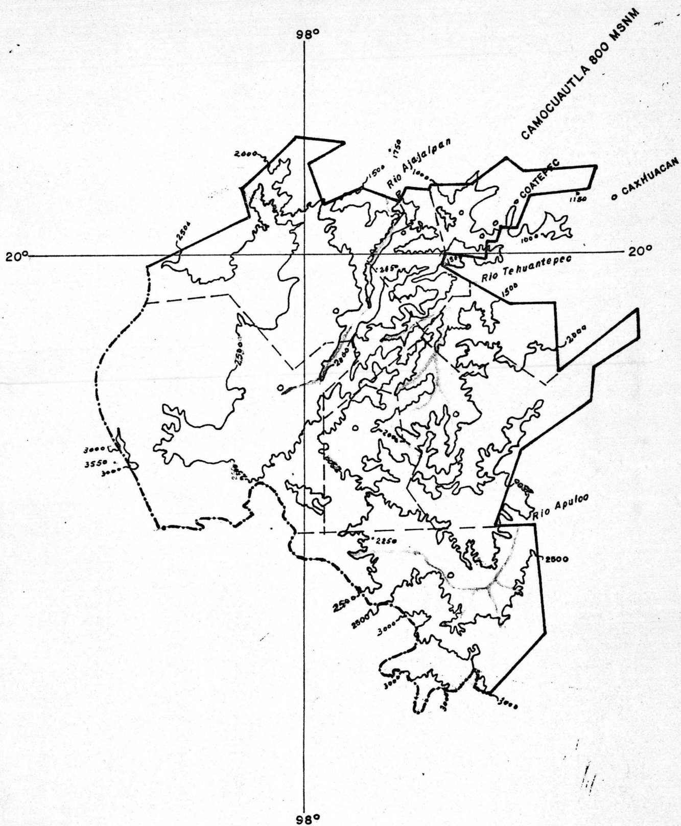
Fig. 2 MAPA TOPOGRAFICO E HIDROLOGICO
