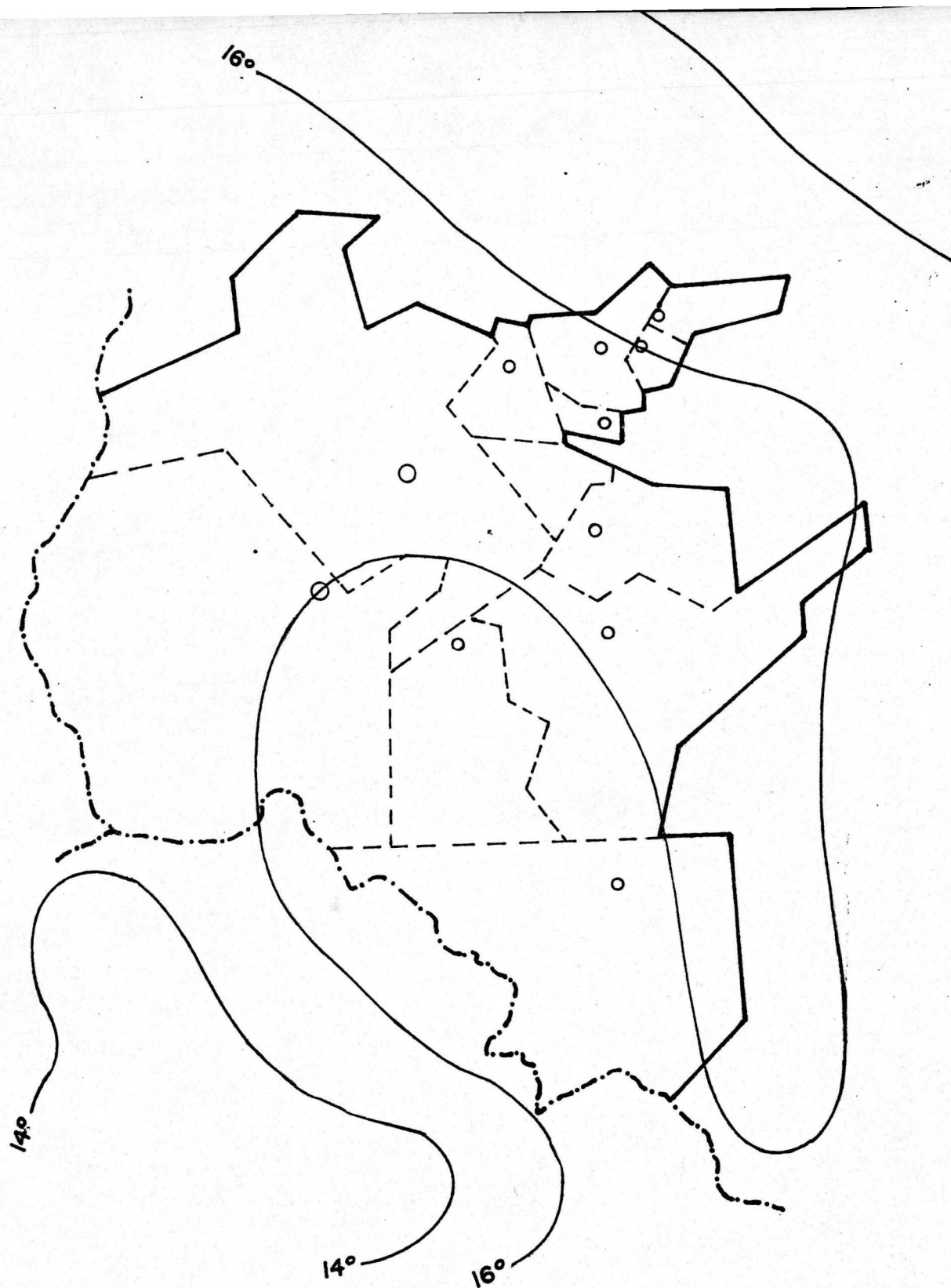
Fig. 3 DISTRIBUCION DE LA TEMPERATURA MEDIA ANUAL (Jáuregui O.E. 1968. mesoclima de la region Puebla-Tlaxcala INSTITUTO DE GEOGRAFIA, UNAM, MEXICO.)
