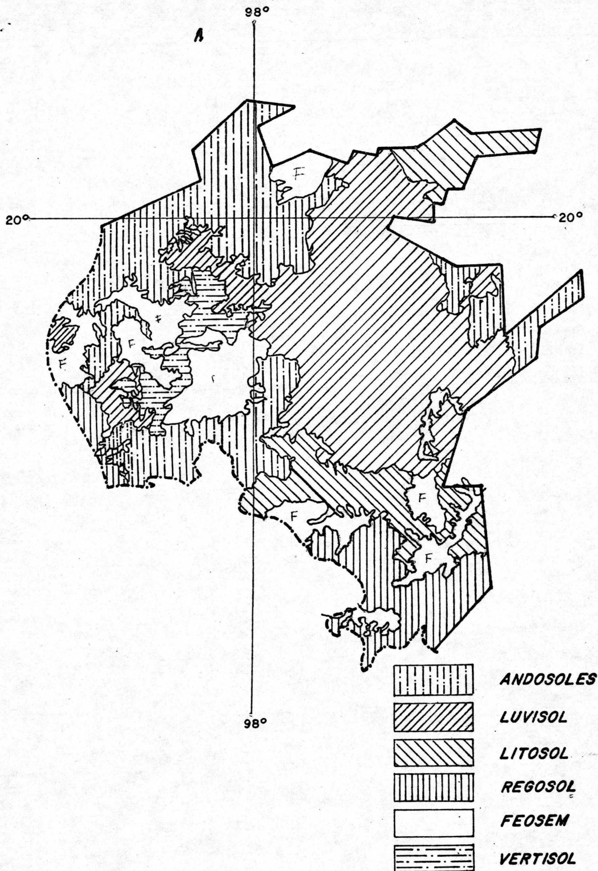
Fig. 6 MAPA DE SUELOS
